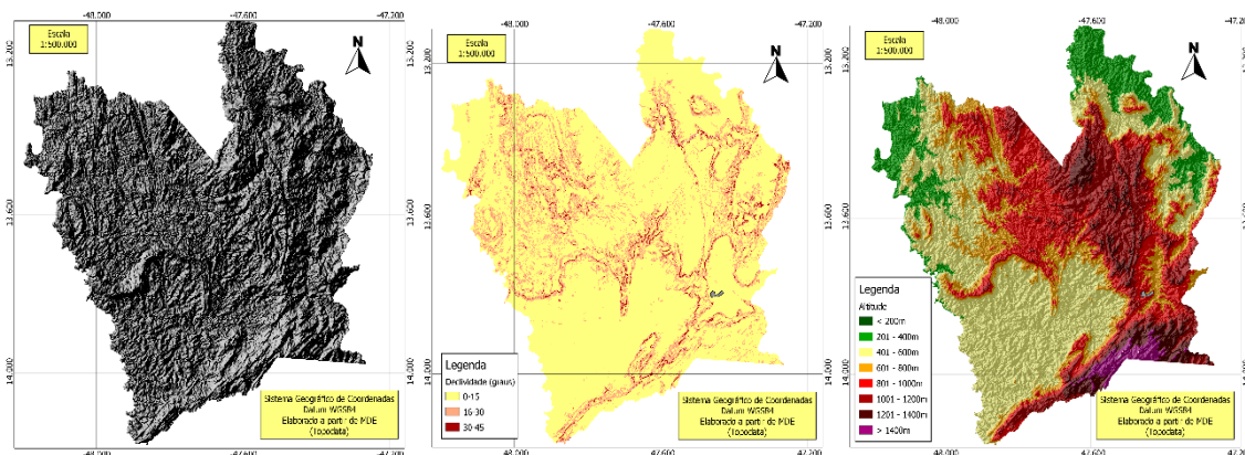
Figura 4. Mapas de relevo sombreado (esquerda), declividade (centro) e hipsométrico (direita) do município de Cavalcante, GO, elaborados e analisados como estudos prévios à aula de campo.
