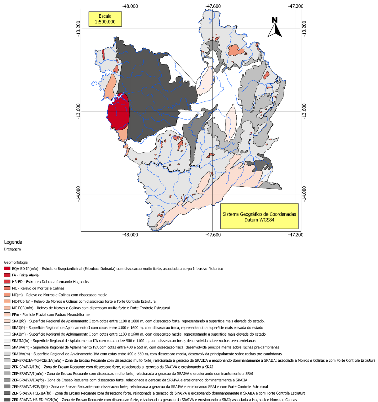
Figura 3. Mapa de unidades geomorfológicas do município de Cavalcante, GO, elaborado e analisado como estudo prévio à aula de campo.
